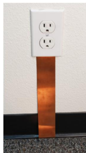
81524 接地用銅板
